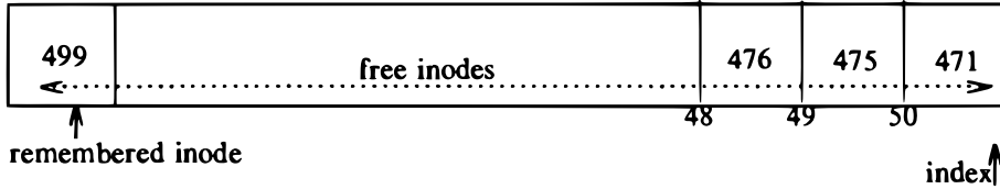
(b) Free Inode 499
