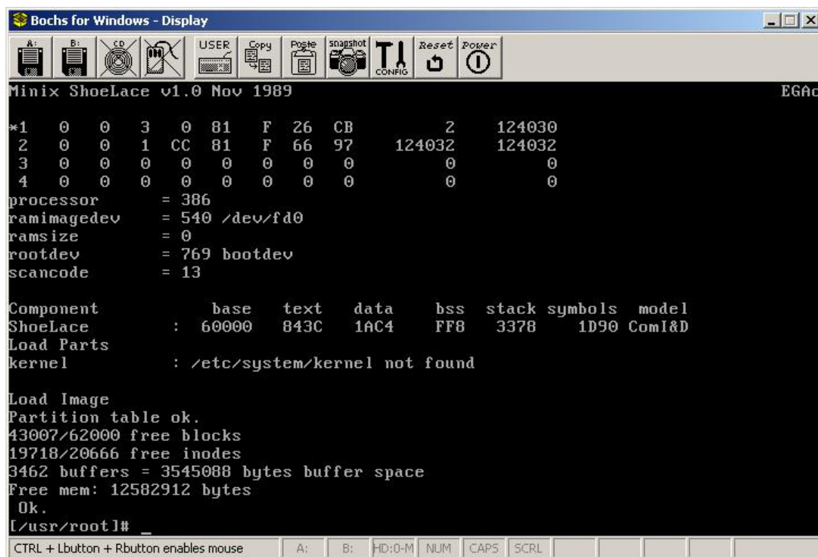
图 17-14 利用 shoelace 从硬盘引导启动 Linux 0.11 系统
