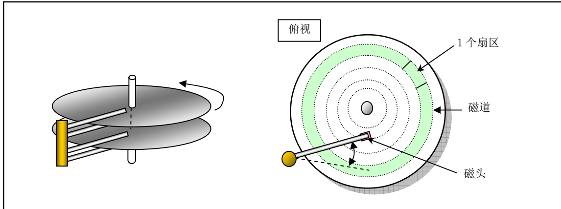
图 2-11 具有 2 张盘片的典型硬盘内部结构
